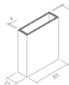
SEZIONE PROFILO
