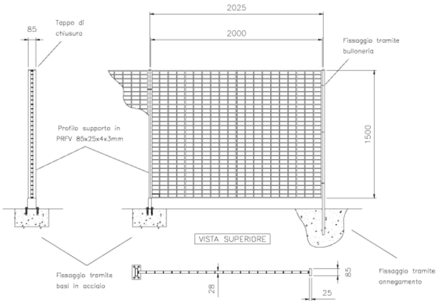
VISTA LATERALE
