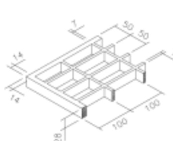
DETTAGLIO GRIGLIATO
